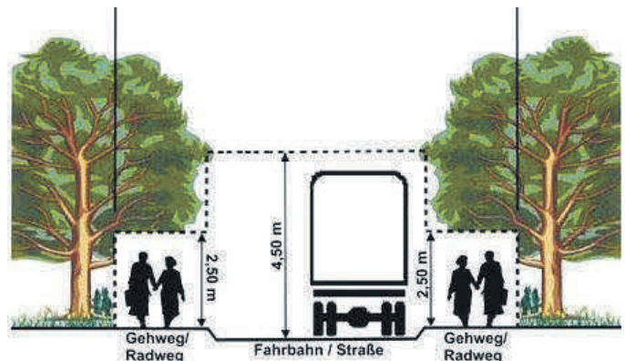
Abb.: Das Lichtraumprofil an öffentlichen Straßen und Geh- bzw. Radwegen.
