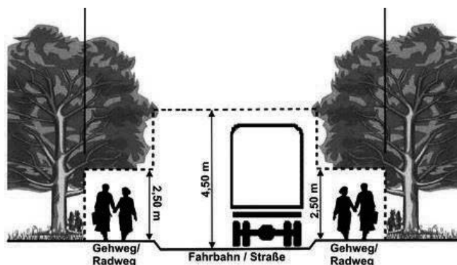
Abb.: Das Lichtraumprofil an öffentlichen Straßen und Gehwegen.
